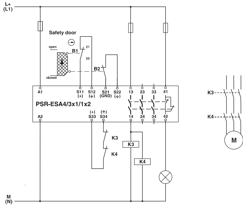
电路图
