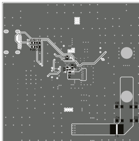
Bottom Layer
