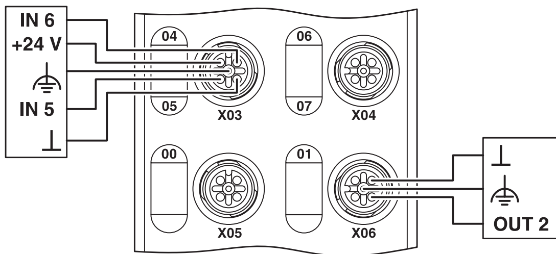
接线图
