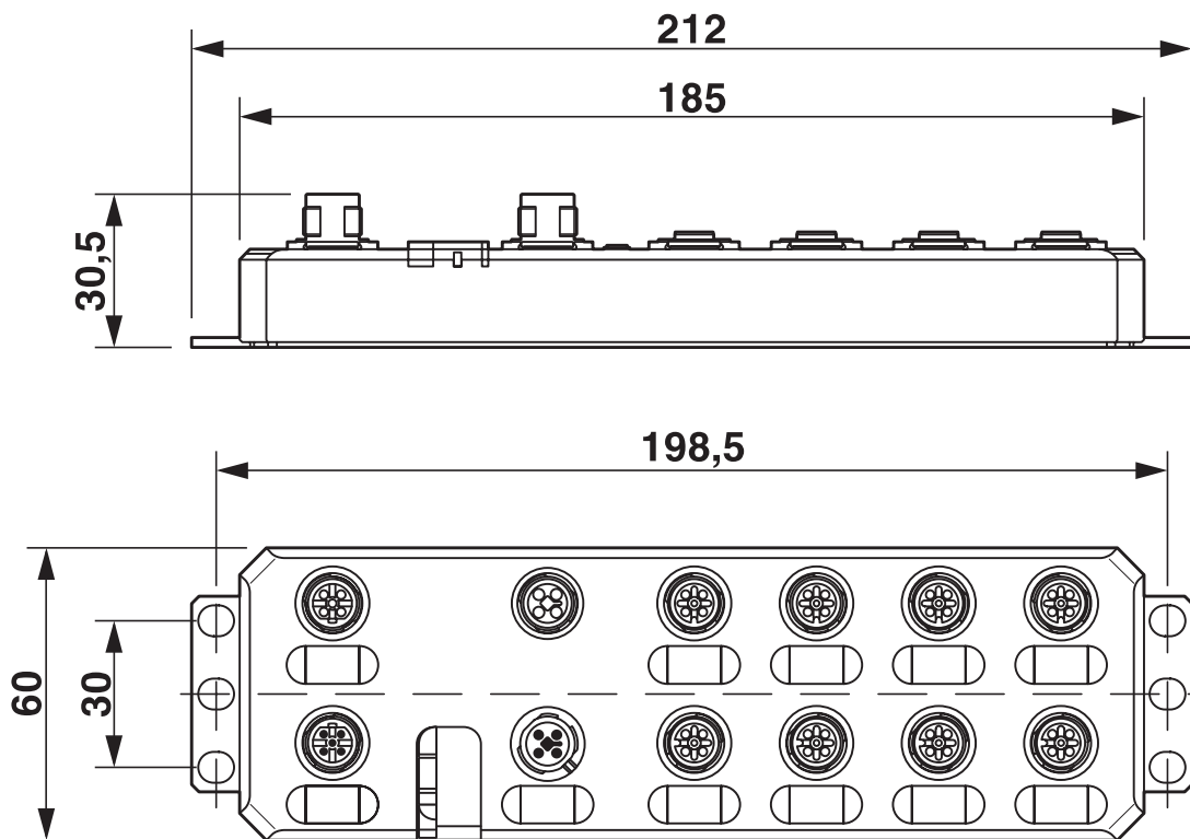
尺寸图
