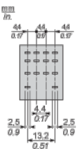
Stecker-Seitenansicht
