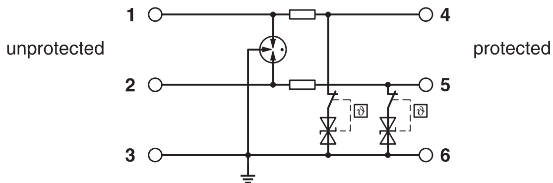
电路图
