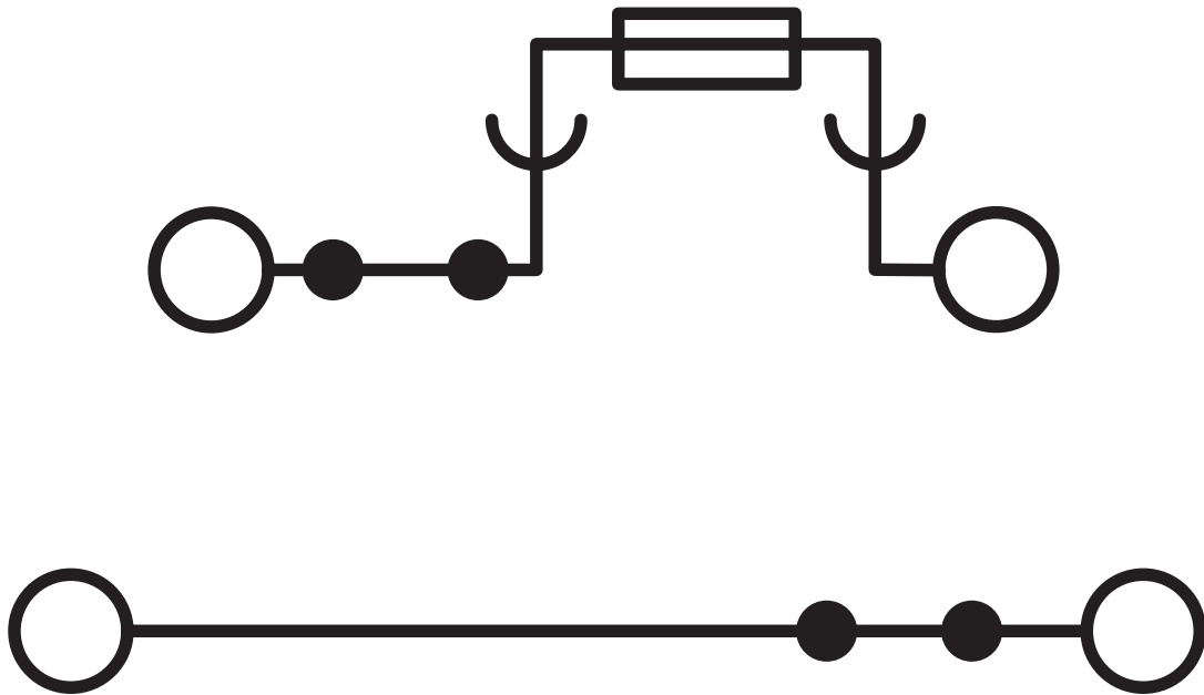
电路图
