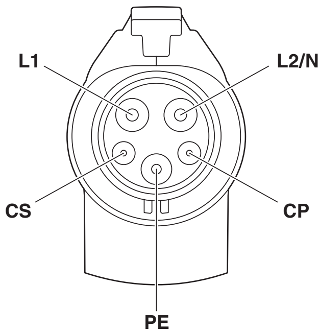
接线图
