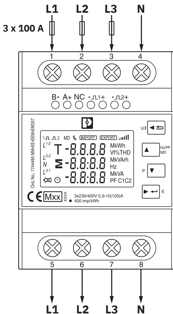
Dessin schématique
