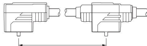
外形寸法
