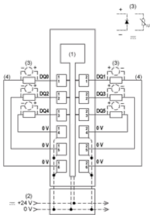
接线图
