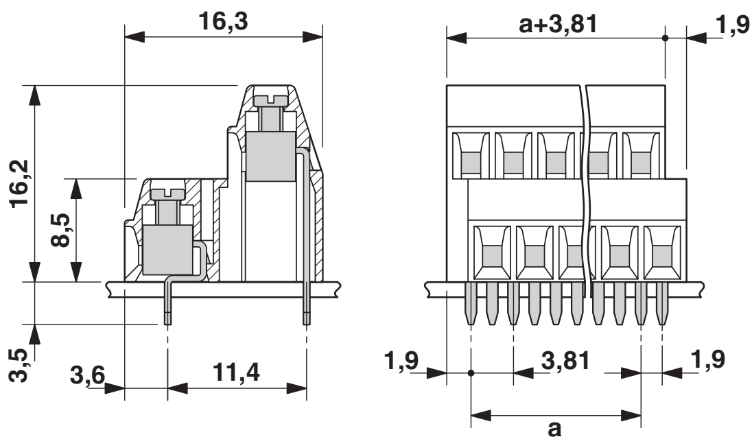
尺寸图
