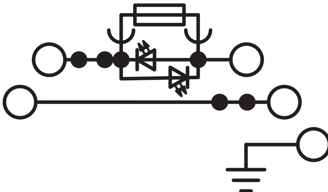
电路图
