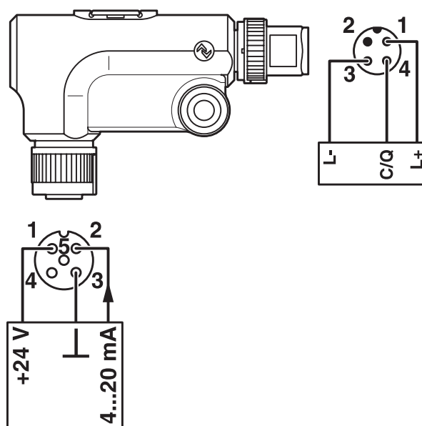
接线图
