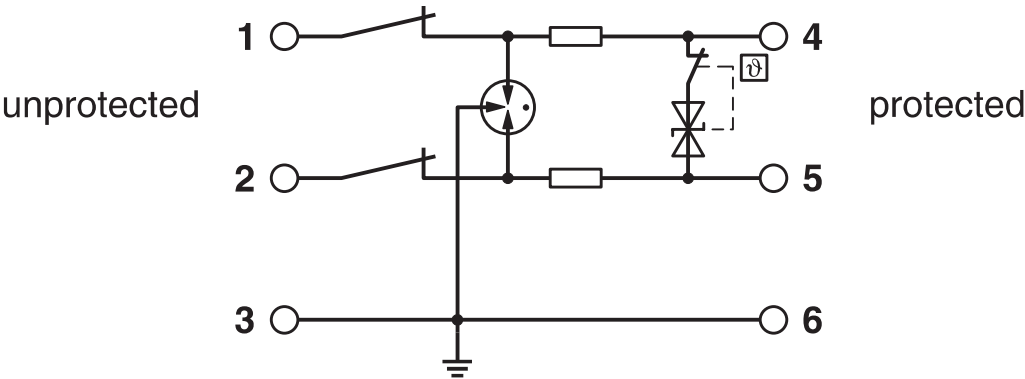
电路图
