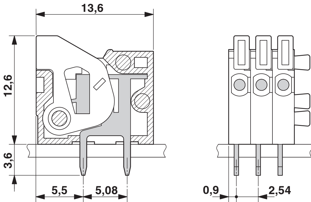
尺寸图
