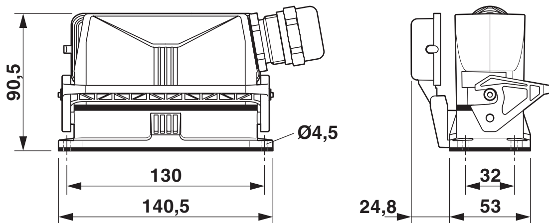
Maßzeichnung
