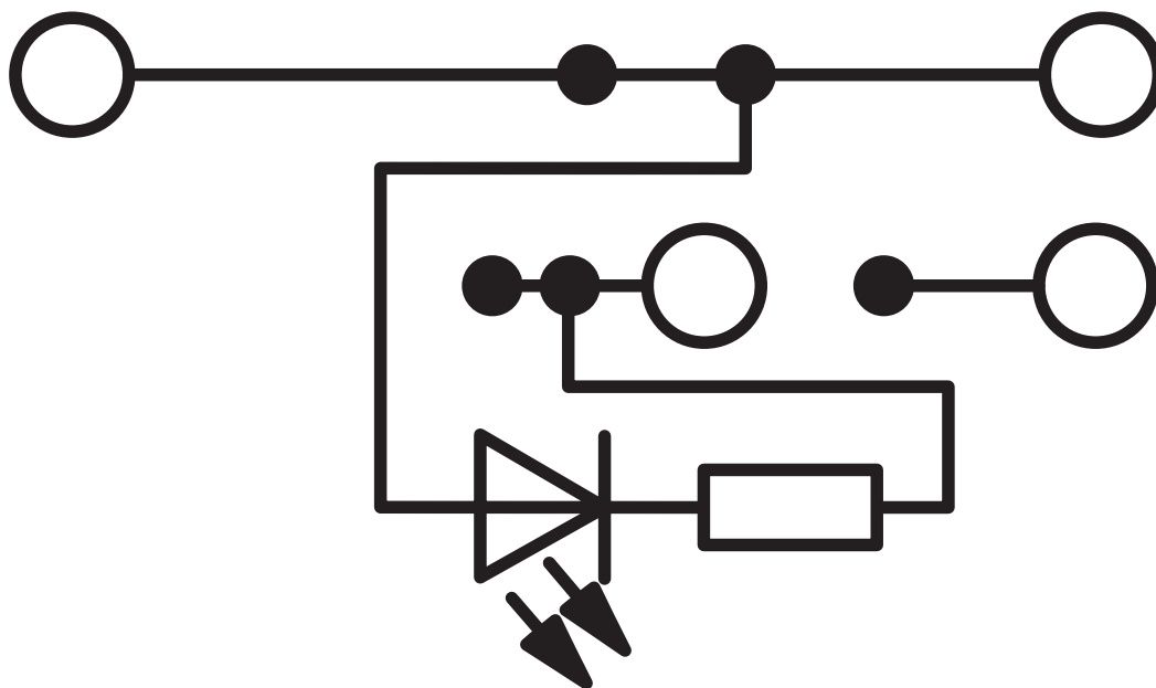
电路图
