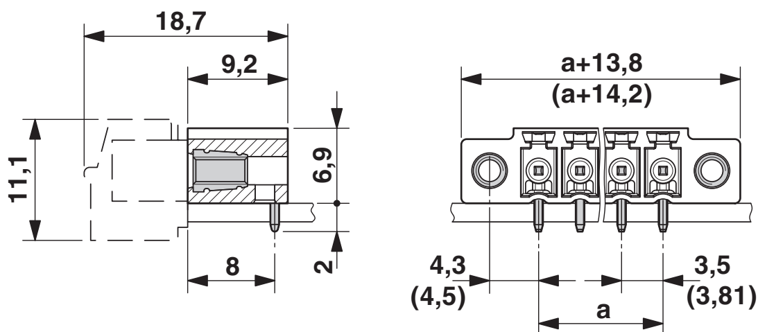
尺寸图
