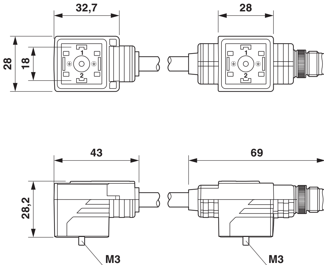
尺寸图
