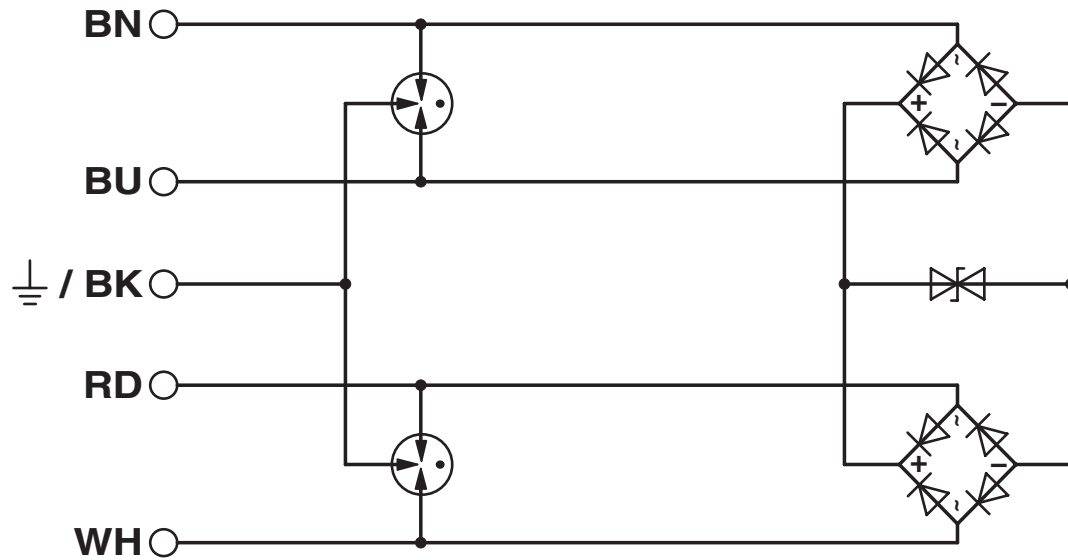
电路图
