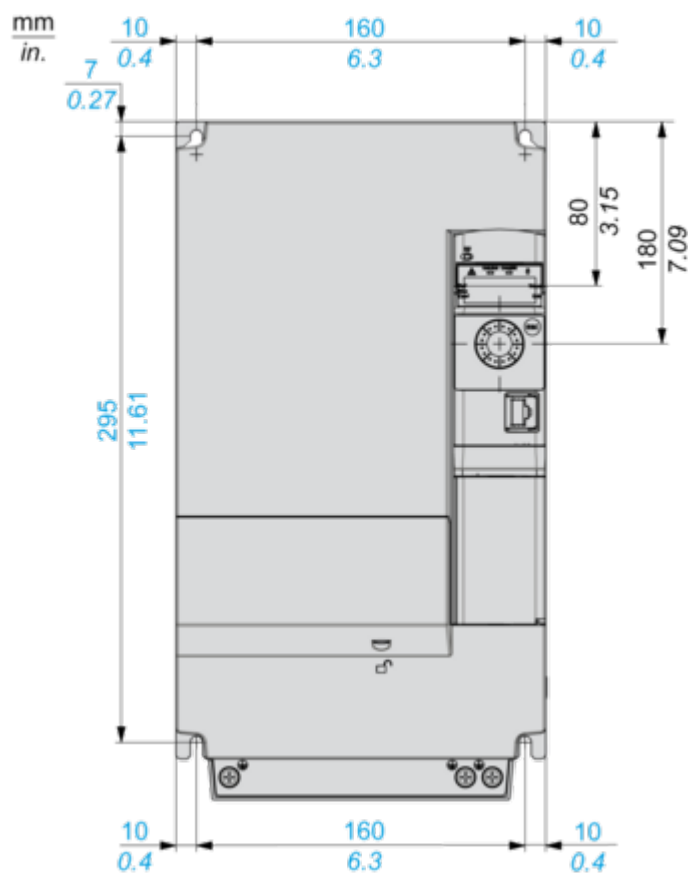
右側视图、正面视图和帶 EMC 板的正面视图
