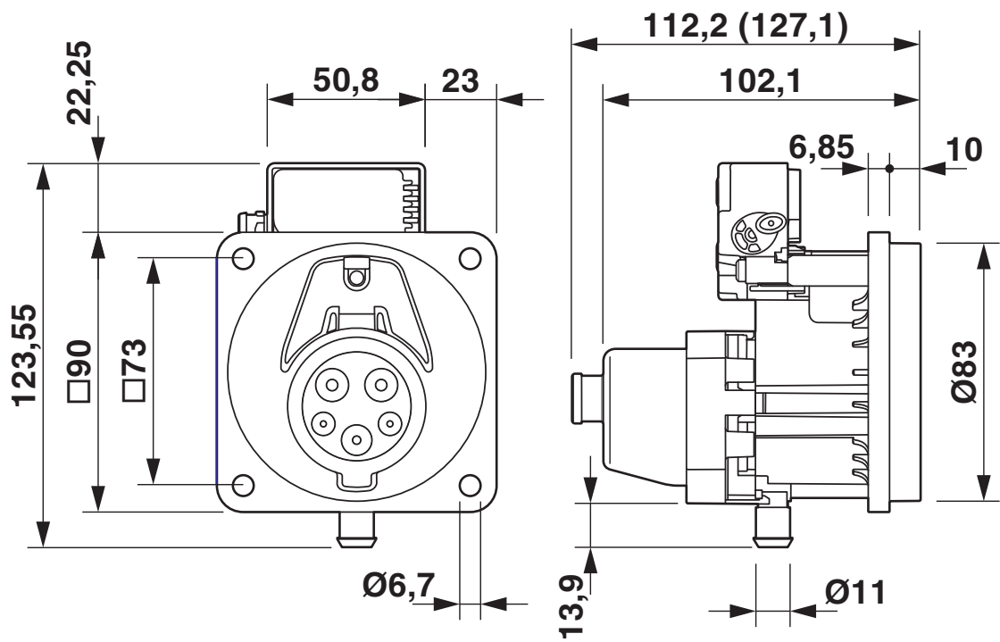
尺寸图
