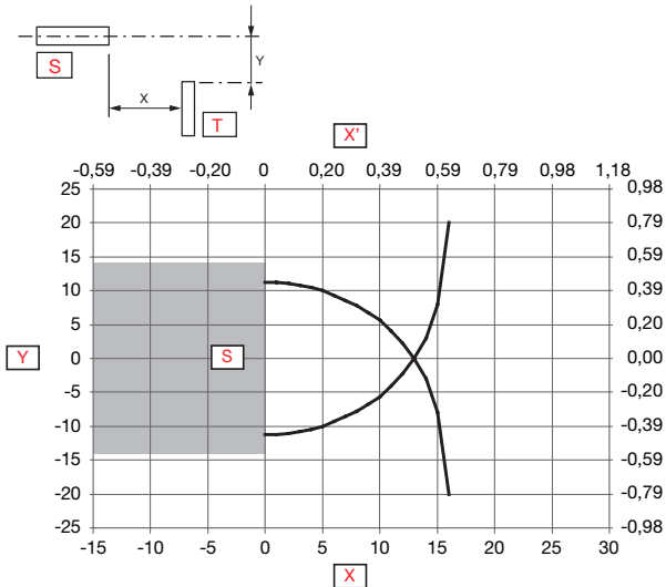
Fig. 4 Affleurant
