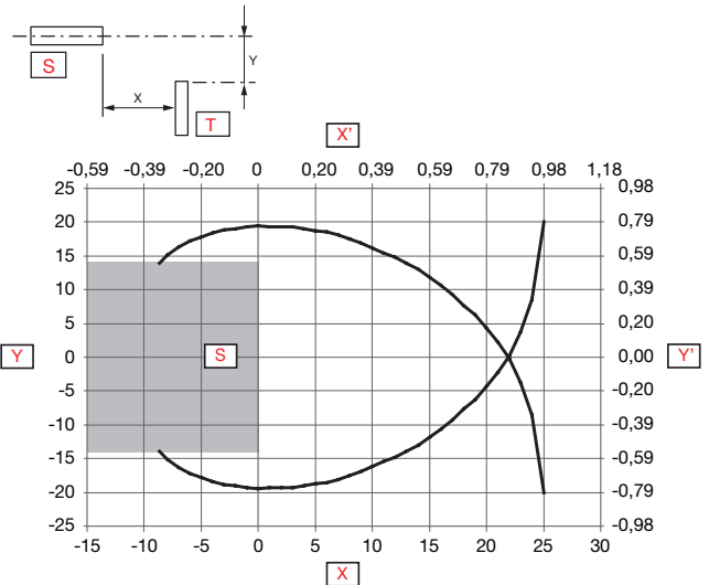
Fig. 5 Non affleurant
