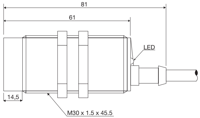
Fig. 7 Câble CA30CAN...A2IO
