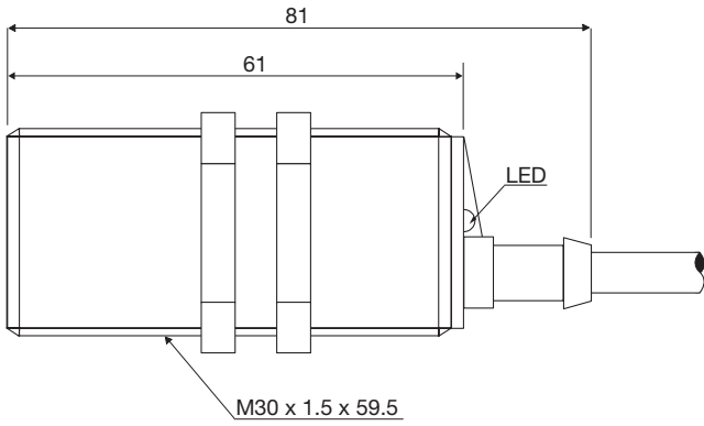
Fig. 6 Câble CA30CAF...A2IO
