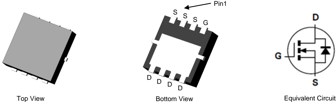
PowerDI3333-8 (Type UX)
