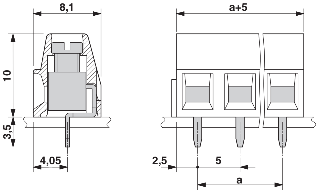
尺寸图
