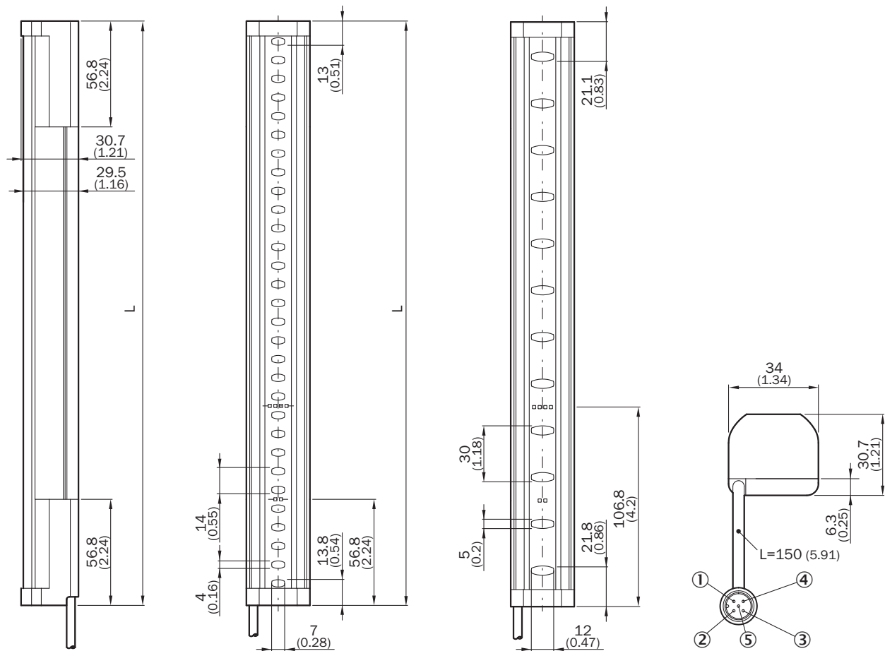
尺寸圖 (尺寸 (mm))
