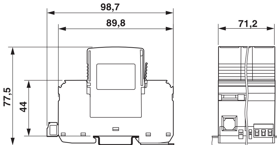
尺寸图
