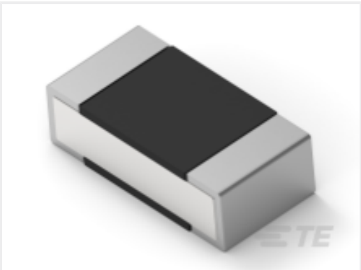
TE Part #5-2176312-3 RP 1E 0.1W 43K2 0.1% 25PPM 1K RL
