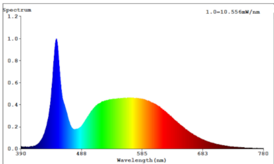
Spektrum
