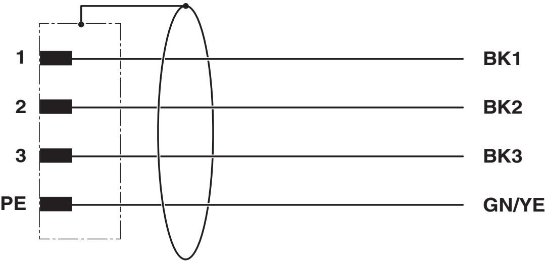
电路图
