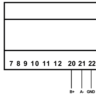
Modbus RTU: RS485 Master
