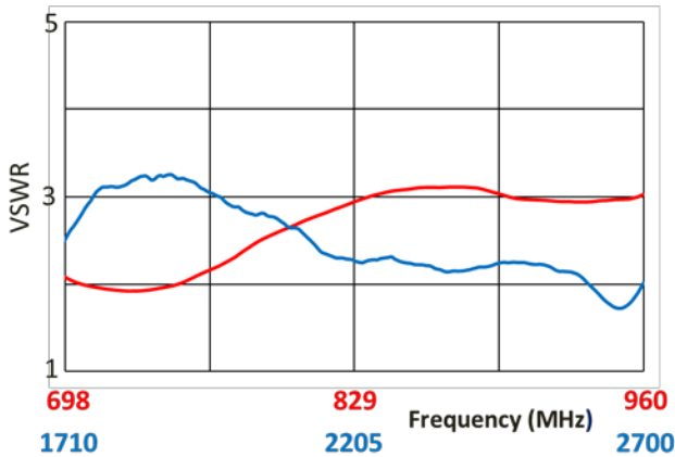
VSWR
