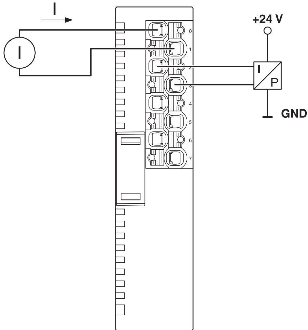
接线图
