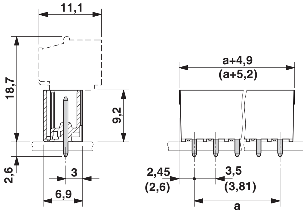
尺寸图
