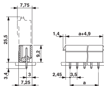
外形寸法
