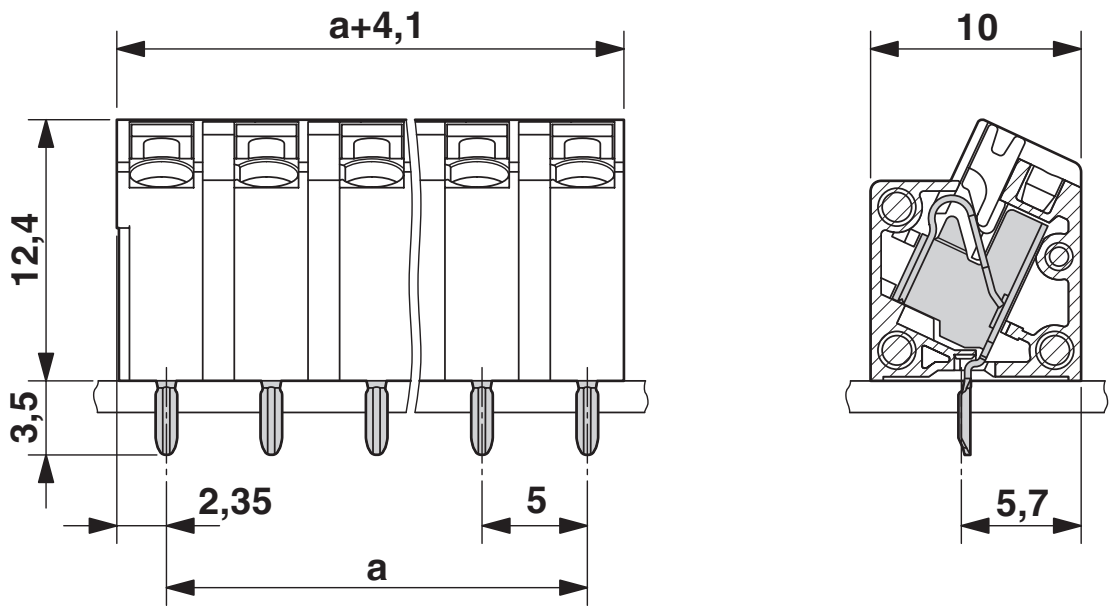
尺寸图
