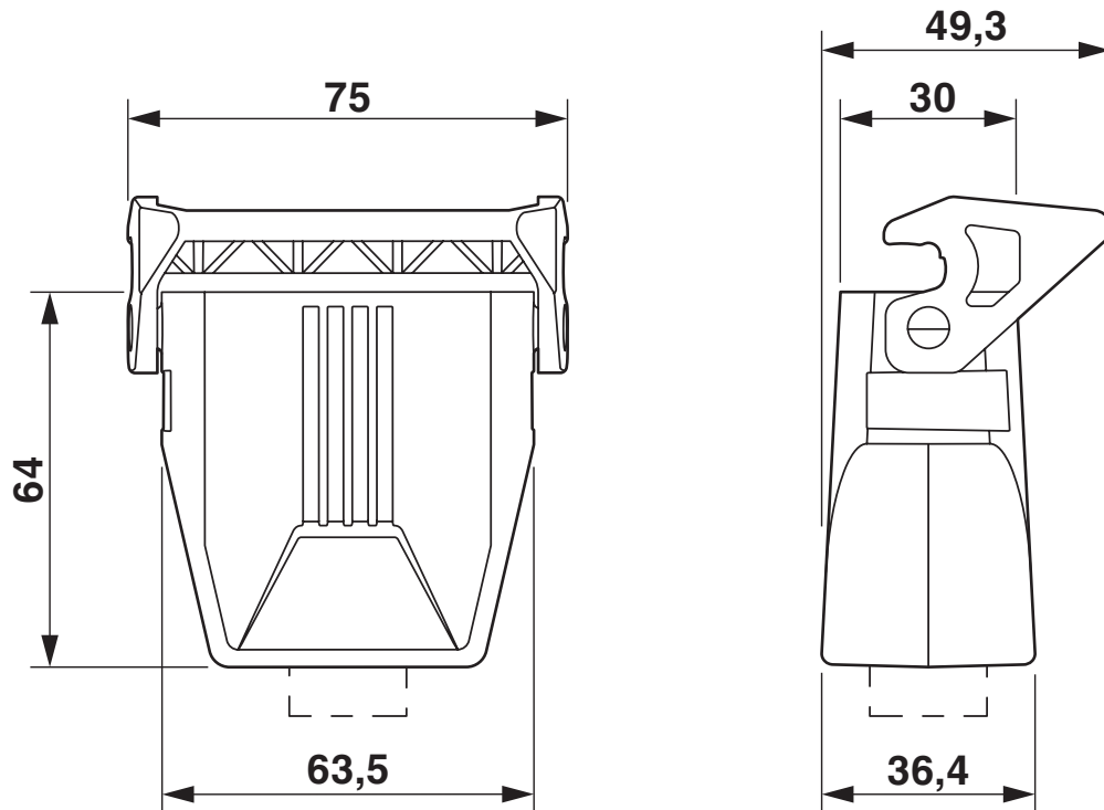
尺寸图
