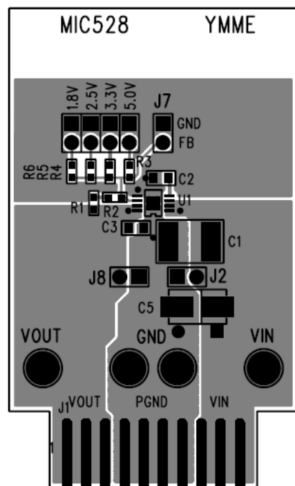
Top Layer Traces
