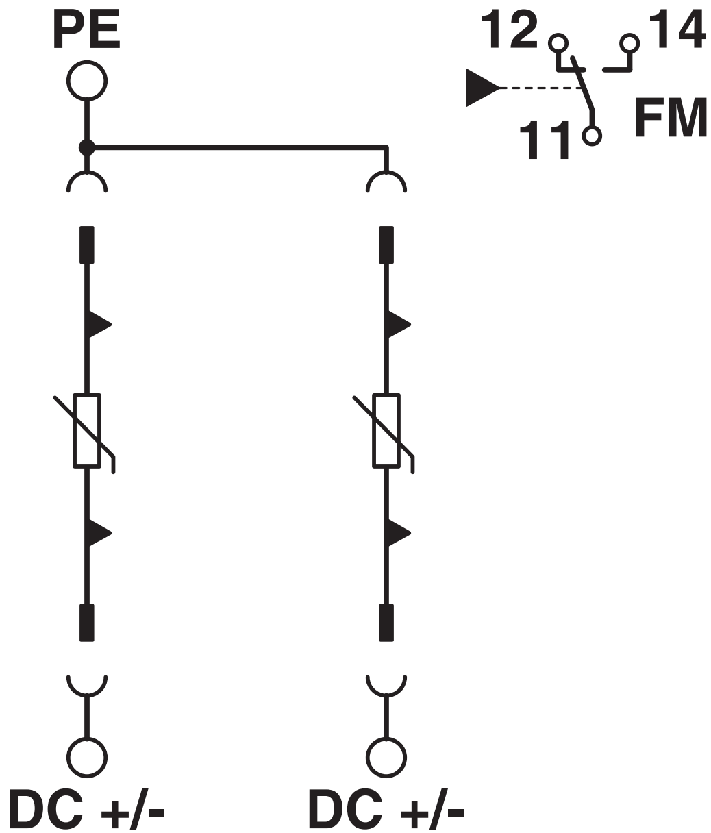
电路图
