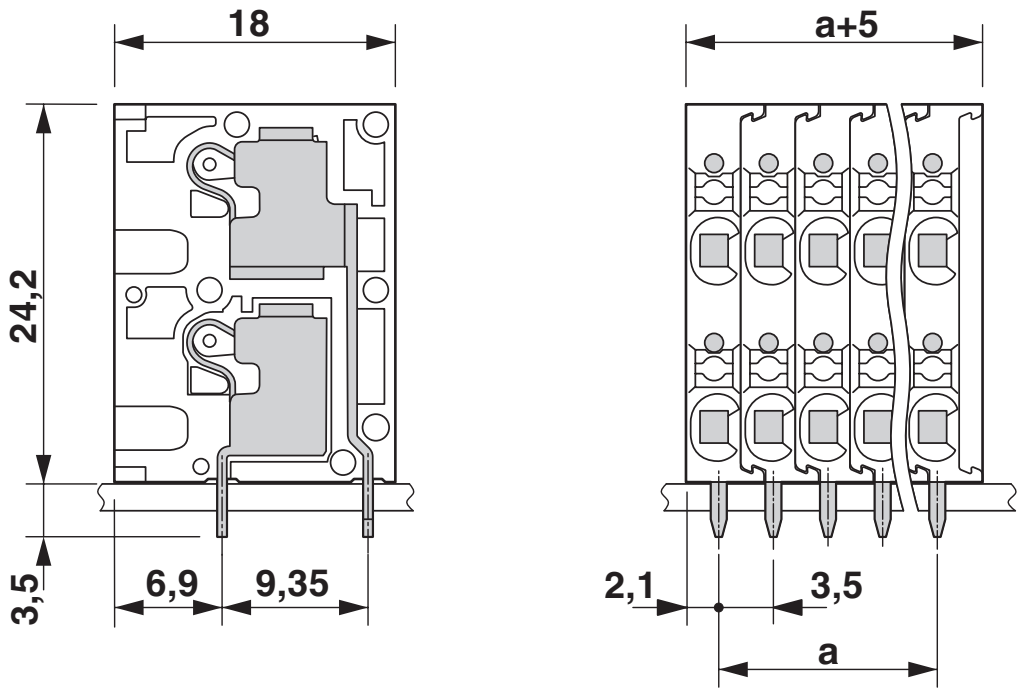
尺寸图
