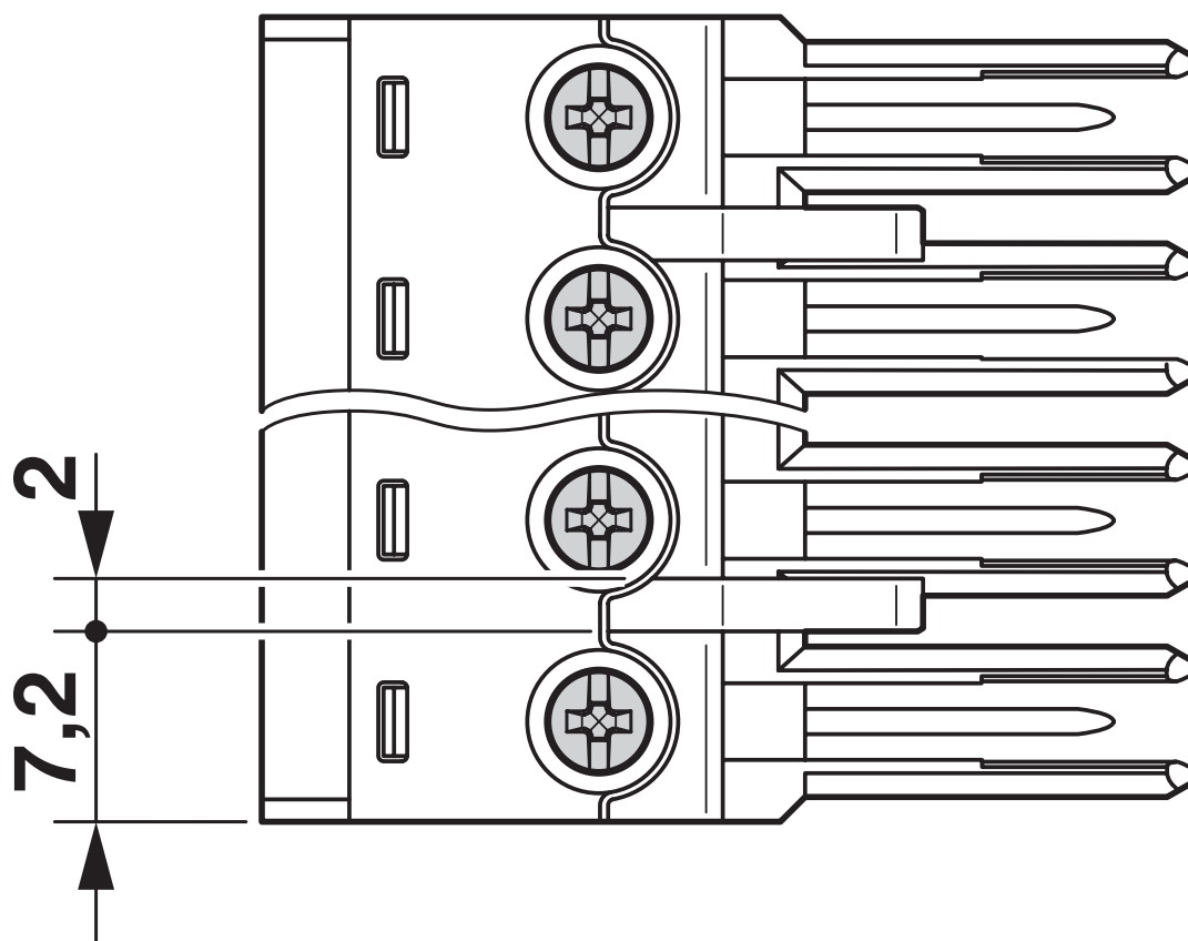
尺寸图
