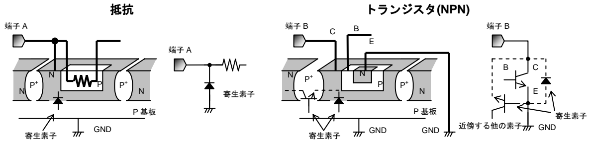
Fig.48 IC の簡易構造例
