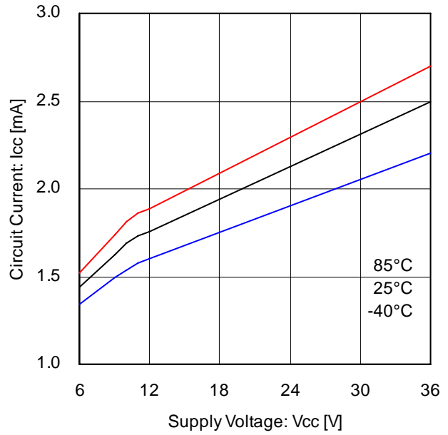
Fig.14 回路電流(2ch)
