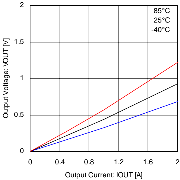
Fig.33 出力 L 電圧(BD6232/37)
