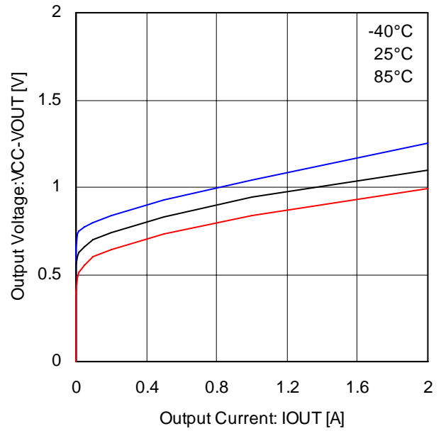
Fig.30 上側 Di 特性(BD6232/37)
