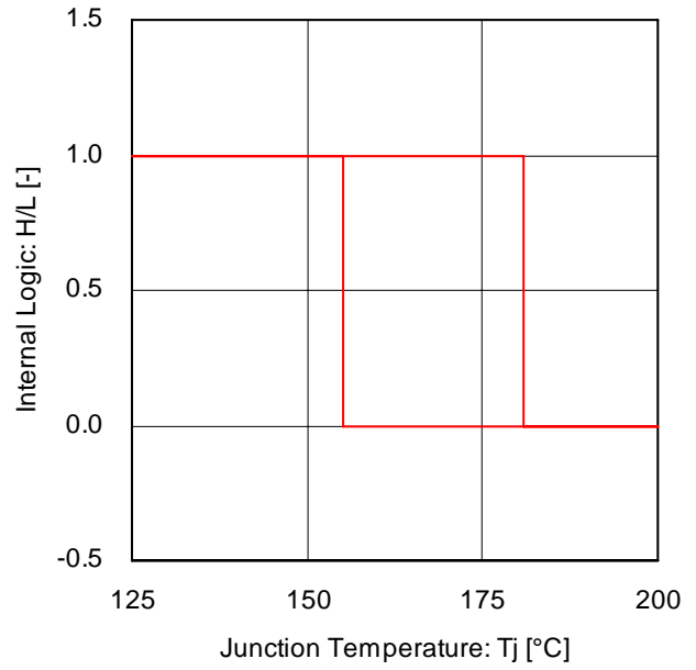
Fig.22 過熱保護回路特性
