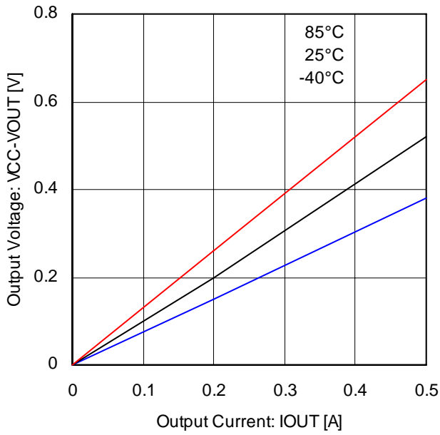
Fig.25 出力 H 電圧(BD6230)
