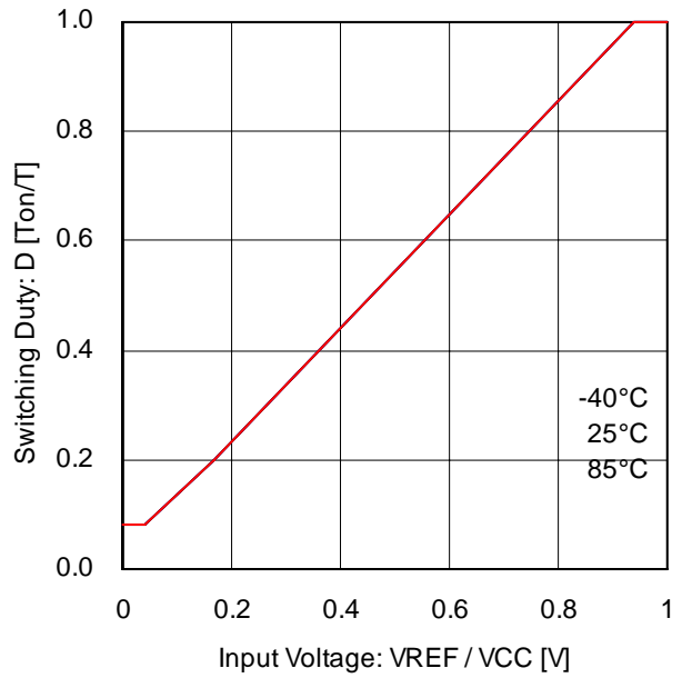
Fig.18 VREF - DUTY 特性 (VCC=24V)
