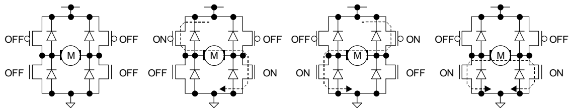
a) スタンバイモード
