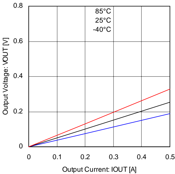
Fig.31 出力 L 電圧(BD6230)
