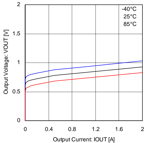
Fig.36 下側 Di 特性(BD6232/37)
