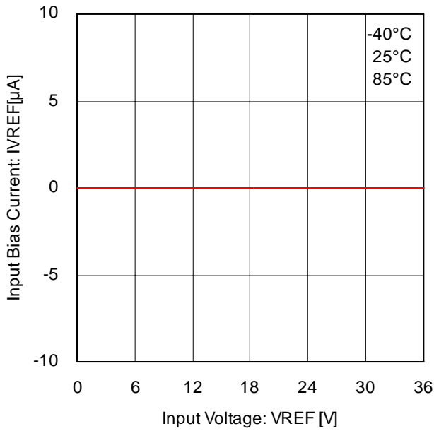
Fig.17 VREF 入力バイアス電流
