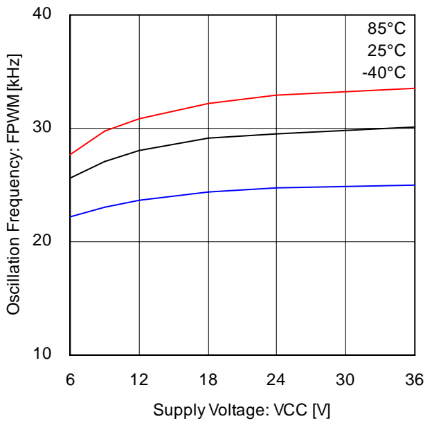
Fig.19 VCC-キャリア周波数特性
