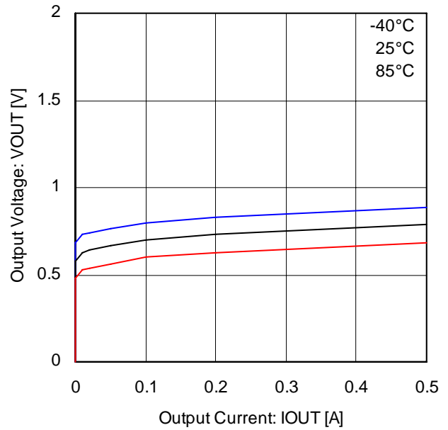
Fig.34 下側 Di 特性(BD6230)
