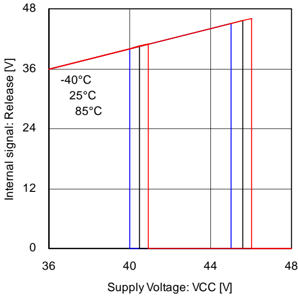
Fig.21 過電圧保護回路特性
