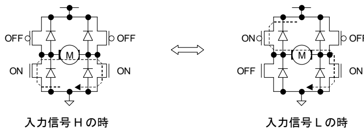
Fig.40 PWM 制御モード(出力)
