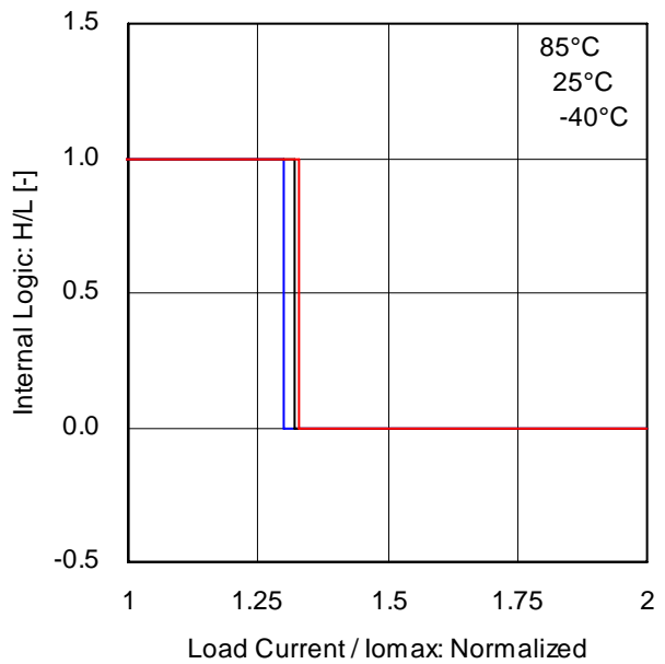
Fig.24 過電流保護回路特性(下)
