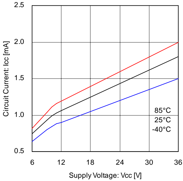
Fig.13 回路電流(1ch)
