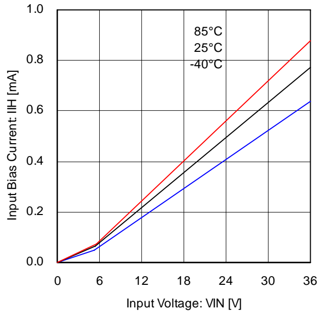
Fig.16 入カバイアス電流
