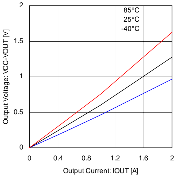
Fig.27 出力 H 電圧(BD6232/37)
