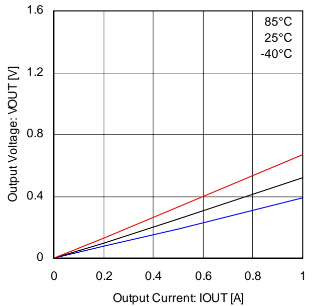
Fig.32 出力 L 電圧(BD6231/36)
