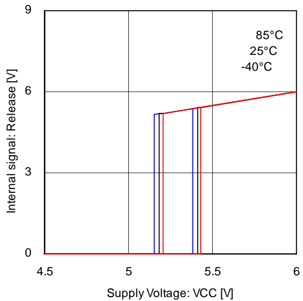
Fig.20 不足電圧保護回路特性
