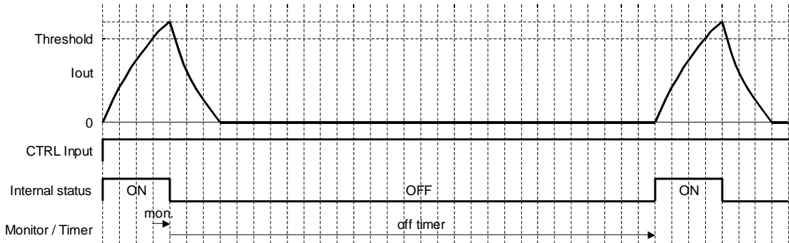
Fig.43 過電流保護動作の例(タイミングチャート)
