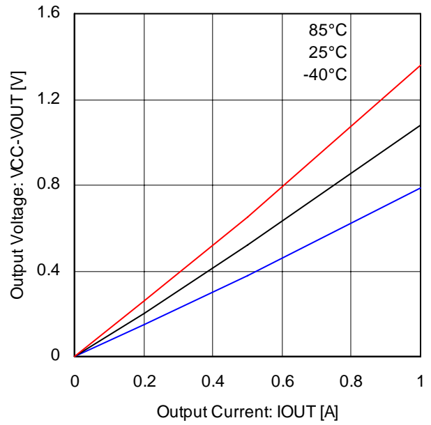
Fig.26 出力 H 電圧(BD6231/36)
