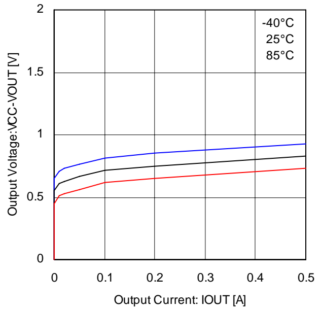
Fig.28 上側 Di 特性(BD6230)
