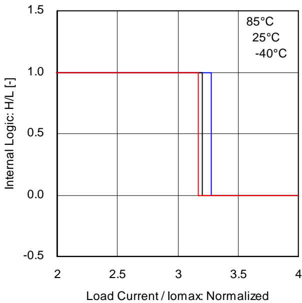
Fig.23 過電流保護回路特性(上)
