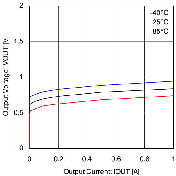
Fig.35 下側 Di 特性(BD6231/36)
