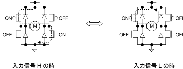
Fig.38 PWM 制御モード(出力)
