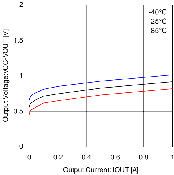
Fig.29 上側 Di 特性(BD6231/36)
