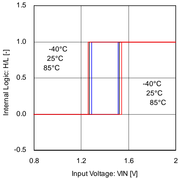
Fig.15 入カスレッシュヨルド電圧
