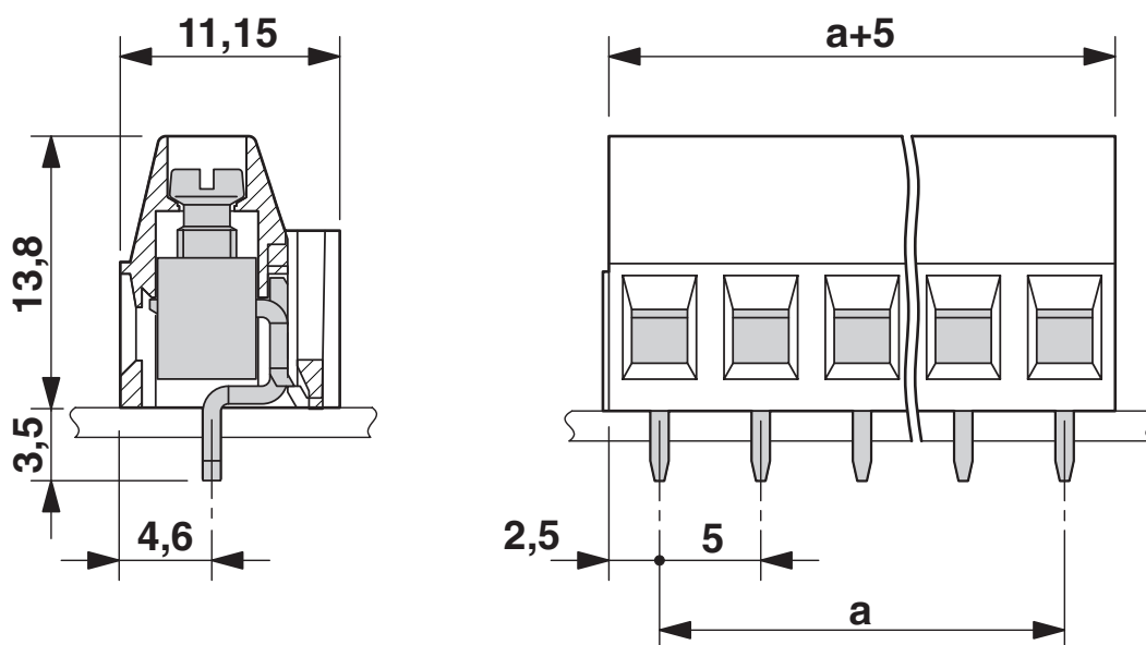
尺寸图
