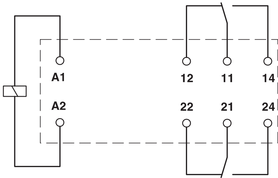
电路图
