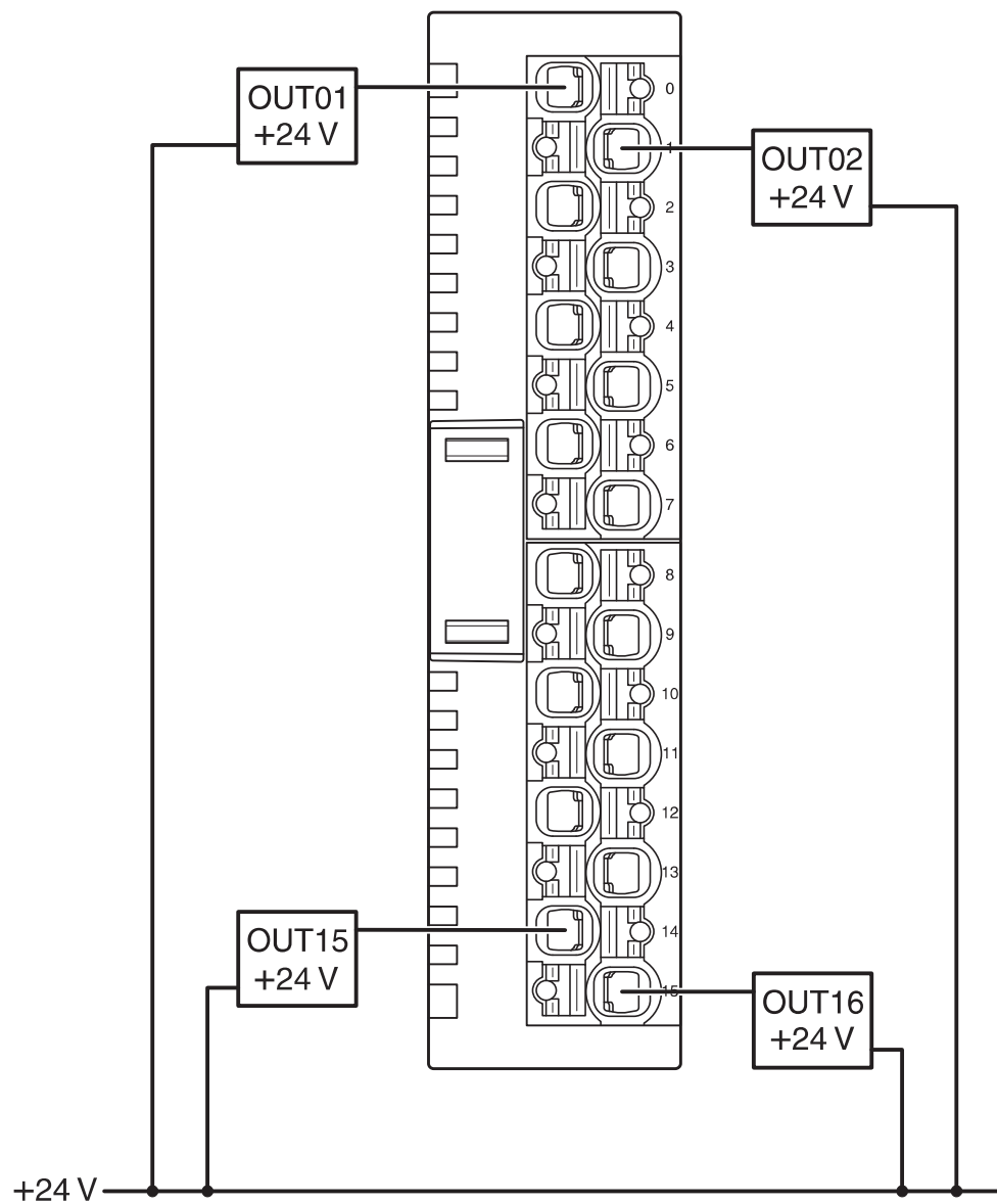
接线图
