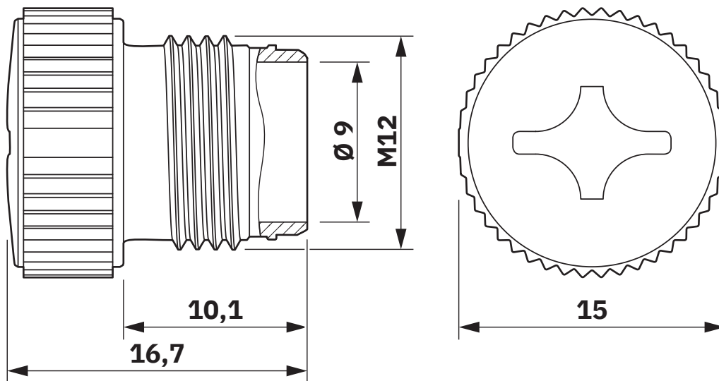
尺寸图
