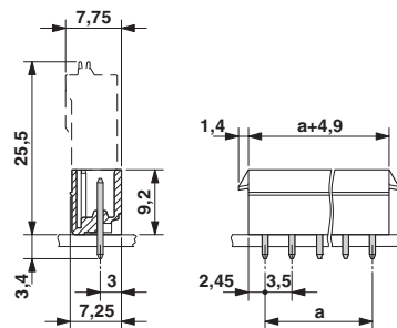
外形寸法
