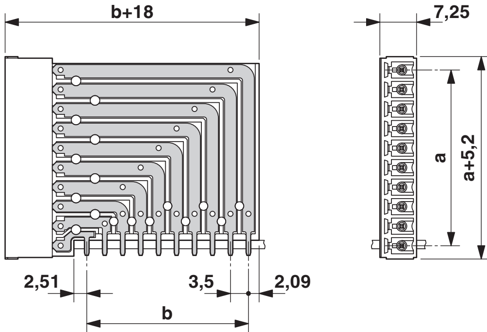
尺寸图
