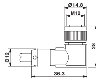
外形寸法
