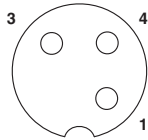
配線図
