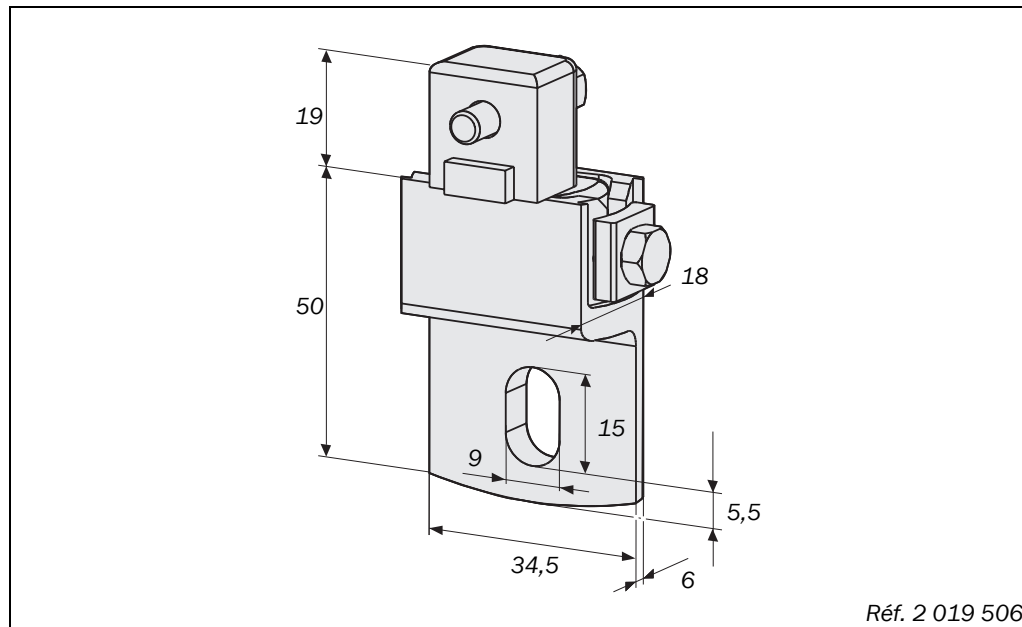
Fig. 28 : Plan coté du support latéral (mm)
