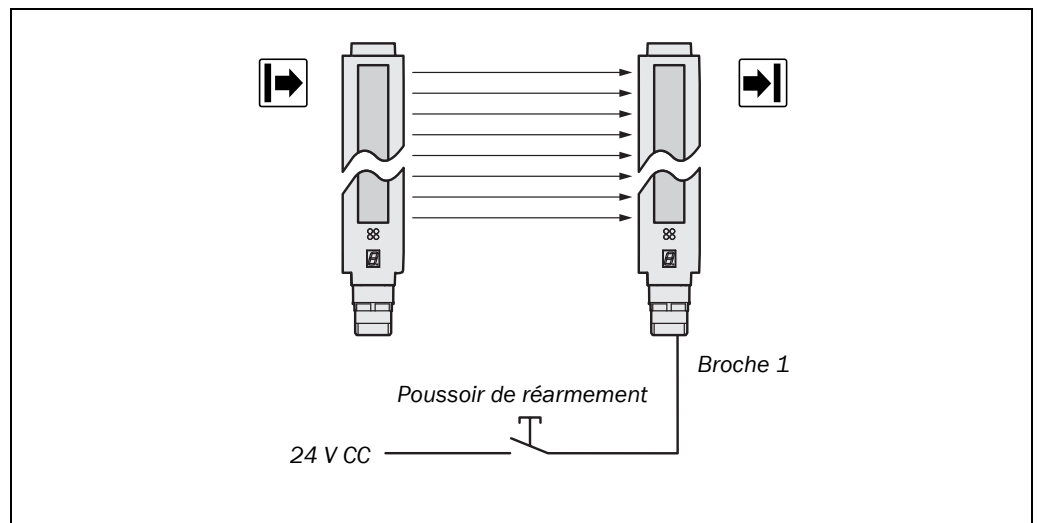
Fig. 21 : Raccordement du pousoir de réarmement au C 4000 Micro
