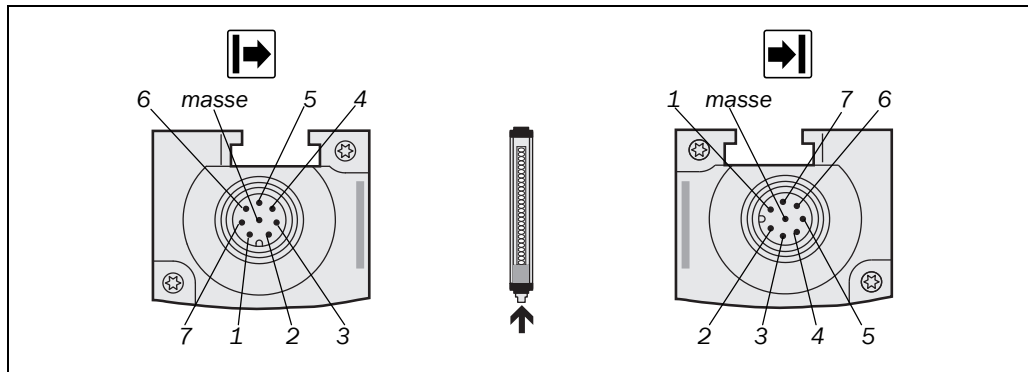
Fig. 19 : Brochage raccordement système C 4000 Micro (M 12×7 + masse)
