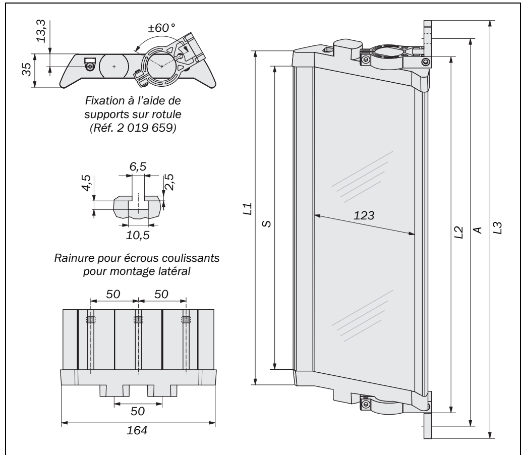
Fig. 30 : Plan coté du miroir de renvoi PNS 125 (mm)
